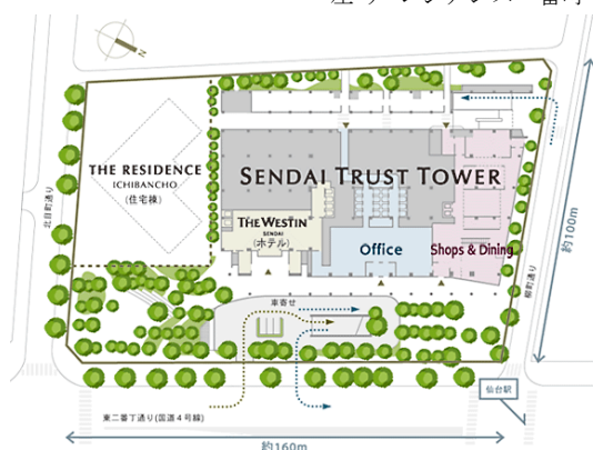
全体配置図
